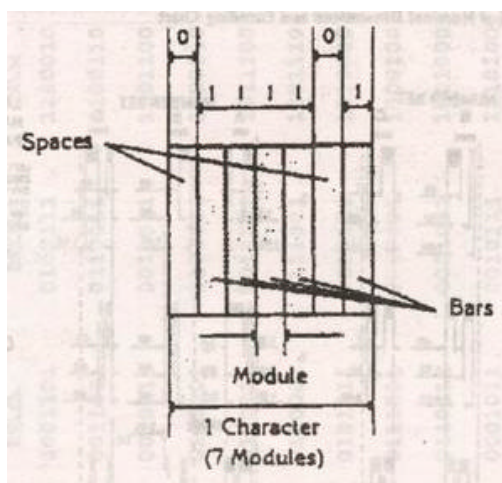
Figura 6 - Modul de alcătuire a unui caracter bar code. Este format din 7 module (bare și spații) care generează 4 alternanțe alb-negru. Un caracter este codificarea grafică a unei cifre zecimale.
