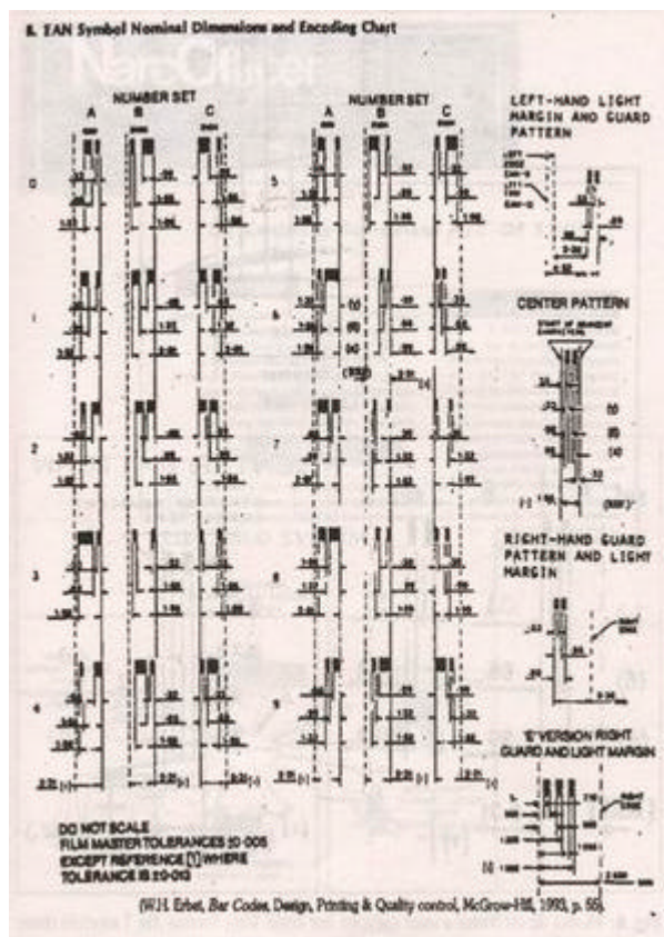
Figura 5 - Tabelul 2 - Dimensiuni nominale și diagrama de codificare a sistemelor EAN. A se urmări îndeosebi compararea măsurătorilor intervalelor specifice pentru cifra 6, și caracterele guard bars (stâng, drept și central)
