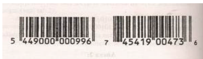
Figura 1 - Etichetele grafice ale tipurilor de cod bară EAN-13 (stânga) și UPC-A (dreapta)
