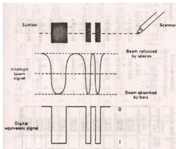
Figura 3 - Modul de generare a semnalelor analogice la trecerea razei laser peste codul barat. Valorile maxime ale semnalului electric generat la citirea unui spațiu determină un semnal digital de valoare 0. Valorile minime ale semnalului electric generat la citirea unei bare determină un semnal digital de valoare 1.
