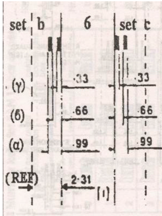
Figurile 7 - Intervalele de citire prin care scannerul generează semnale analogice echivalente la trecerea razei laser peste codul barat. Se observă identitatea mărimilor intervalelor de citire pentru cifra 6 și caracterul guard bar.
